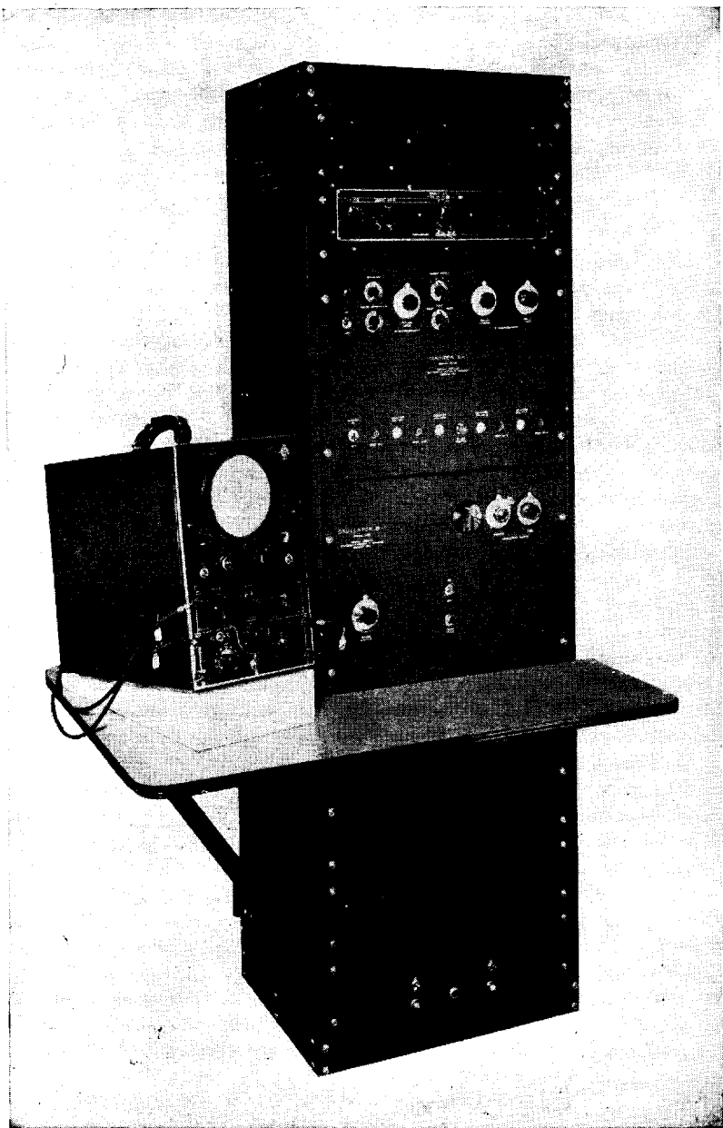
FIG. 7-1.—Model B-1 timer.
