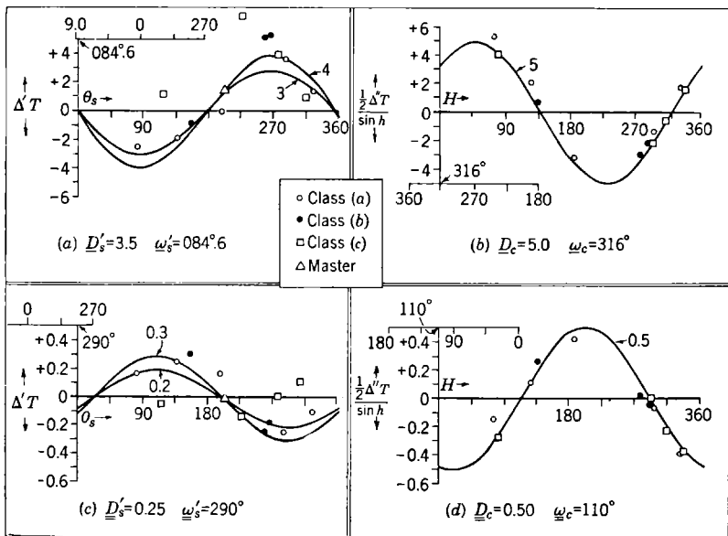
FIG. D-8.—Plots, Example I.
