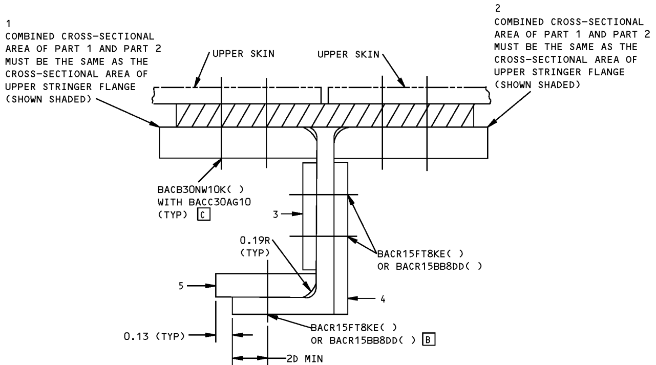
SECTION A-A
