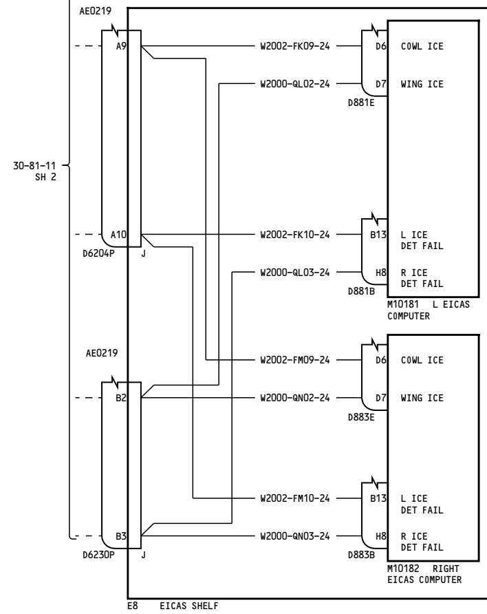
E8 EICAS SHELF
