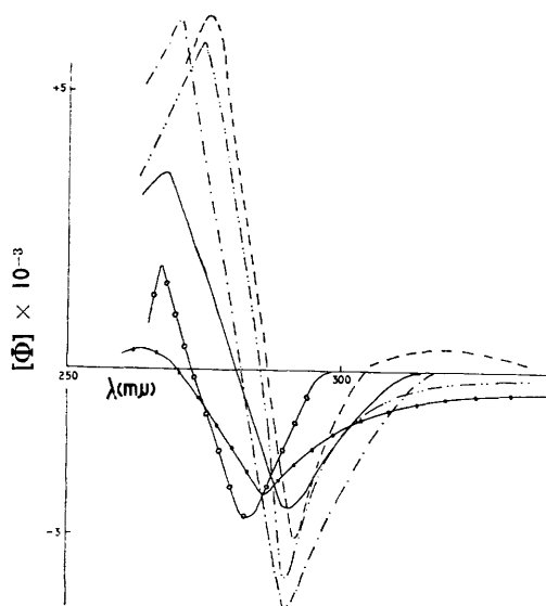
FIGURE 1. Optical rotatory dispersion curves of isoflavans. —●— (—)-Duartin (I); — (—)-mucronulatol (II); — (—) (+)-vestitol (III); —○— (—)-5,7,3',4'-tetramethoxyisoflavan (IV); —·— (—)-equol (VI); —·— (+)-dihydrohomopterocarpin (X).
