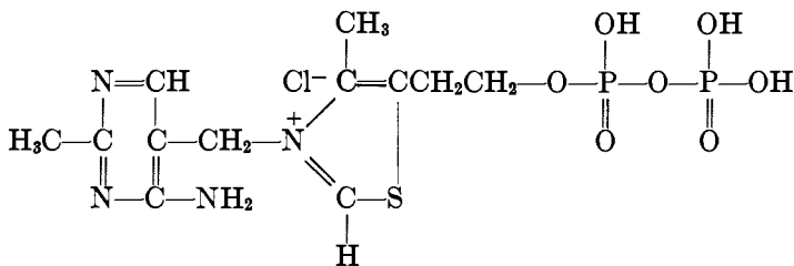
Thiamin nucleotide
