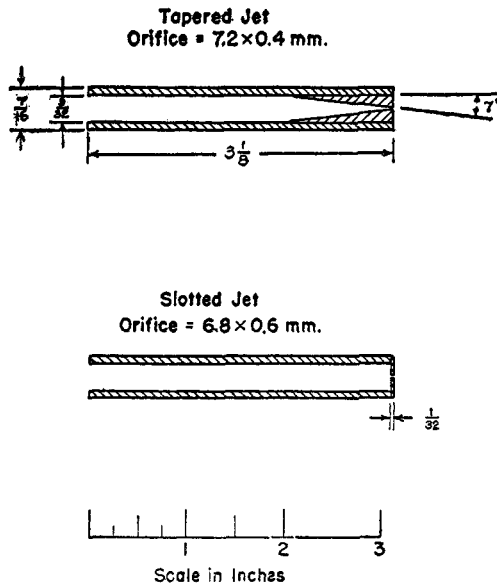
FIG. 6. Impinger jets
