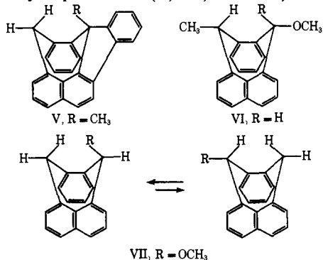
VII, R = OCH 3
