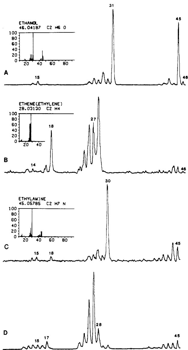
Figure 9. Hg/O 2 NR mass spectra of (A) ionized ethanol, (B) • CH 2 CH 2 O + H 2 , (C) ionized ethylamine, and (D) • CH 2 CH 2 N + H 3 . Inset: EI mass spectra.
