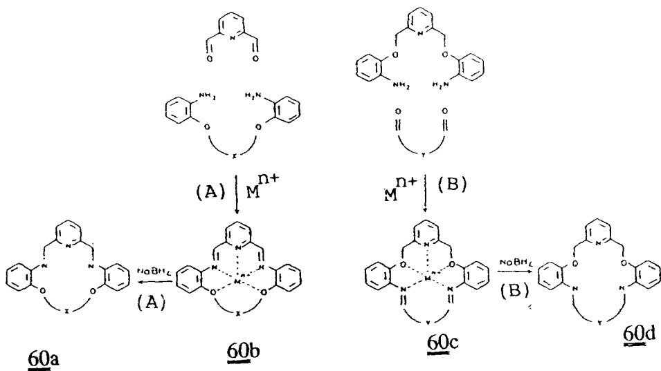
Scheme 21.
