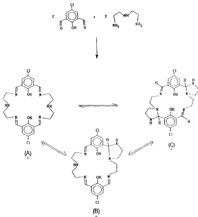
Scheme 16.
