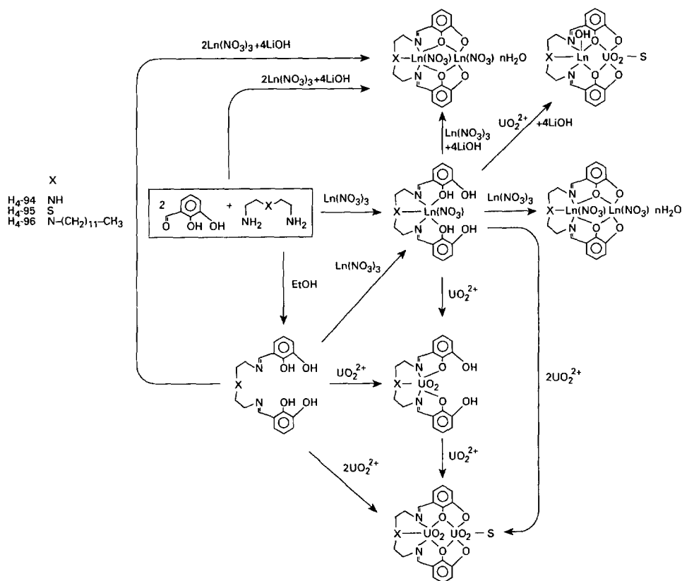
Scheme 31.
