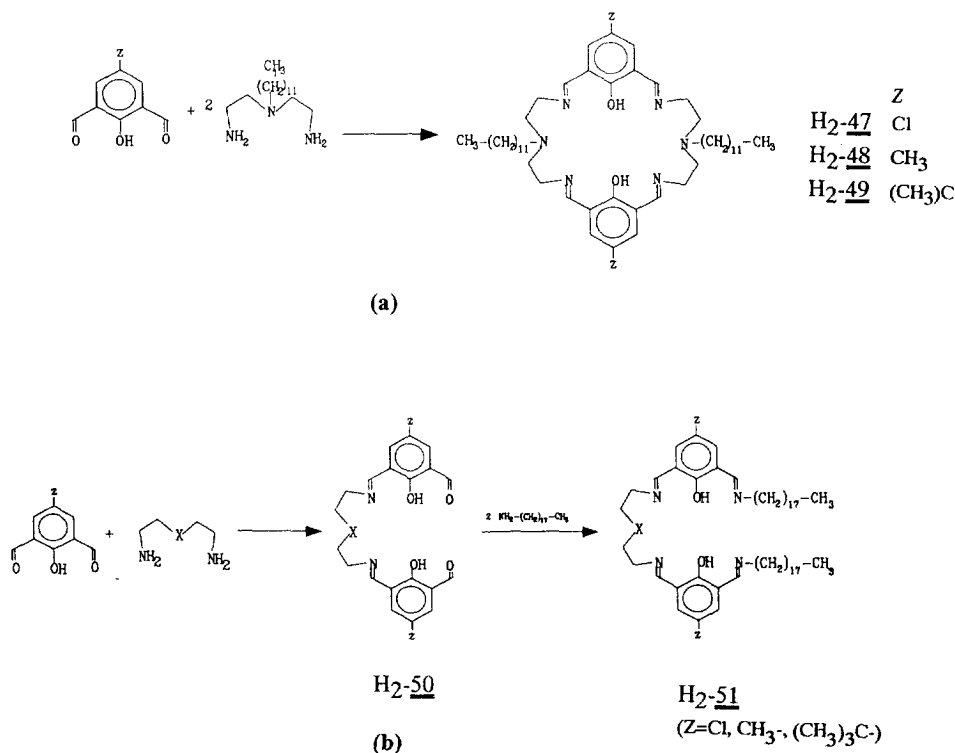
Scheme 19.
