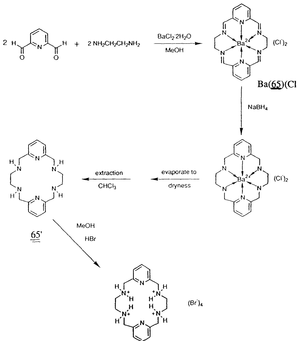
Scheme 24.
