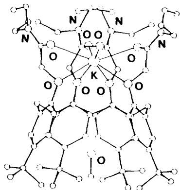
Fig. 6. Structure of \text{K}(\mathbf{10}) \cdot \text{SCN} \cdot \text{MeOH} .
