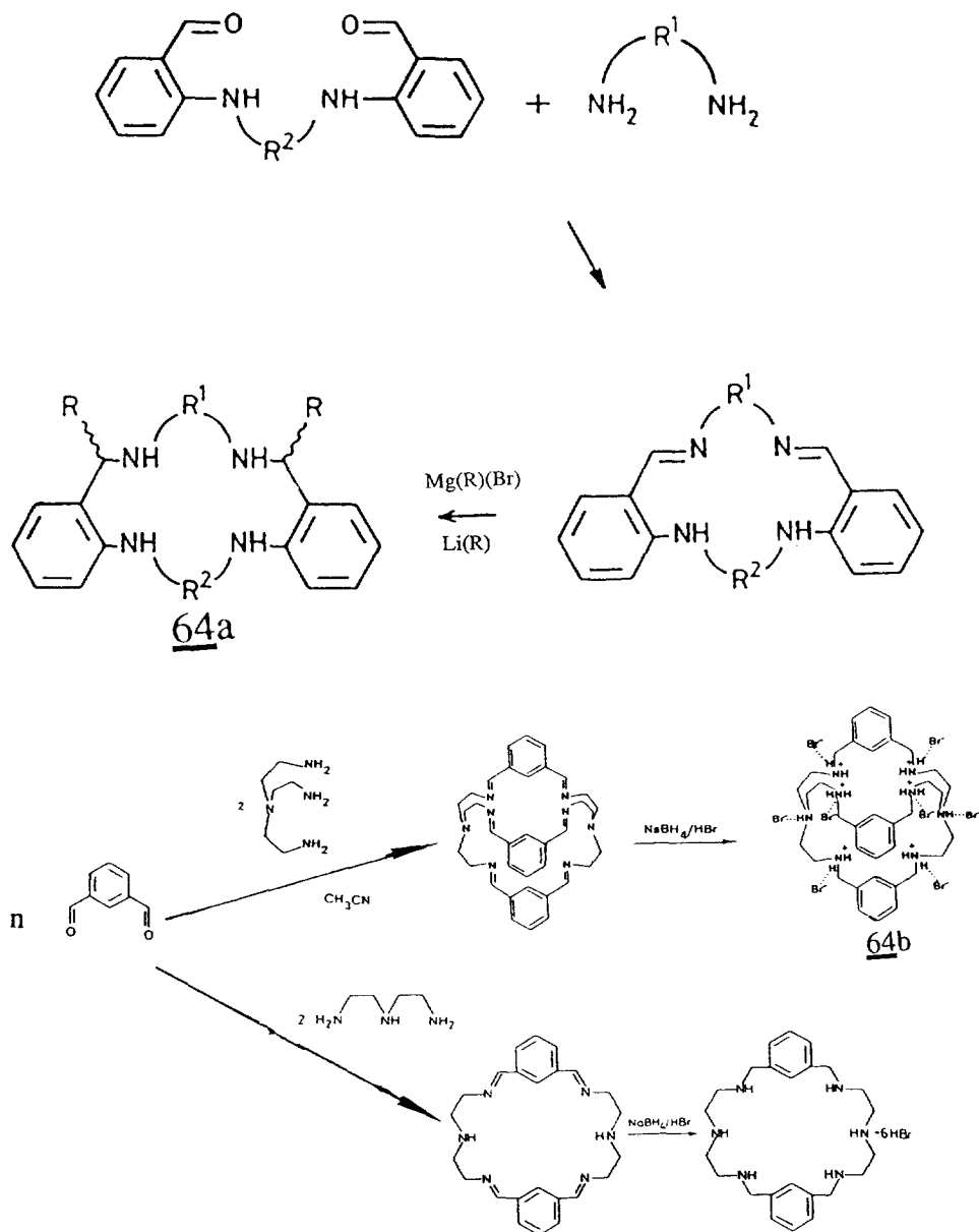
Scheme 23.
