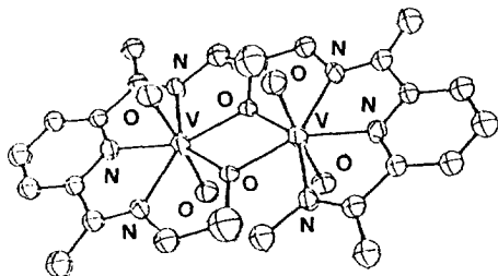
Fig. 31. Structure of [V_2(45-2H)(H_2O)_4]^{2+} .
