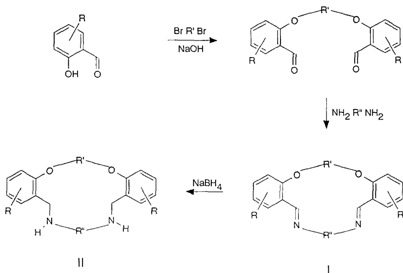
Scheme 22.
