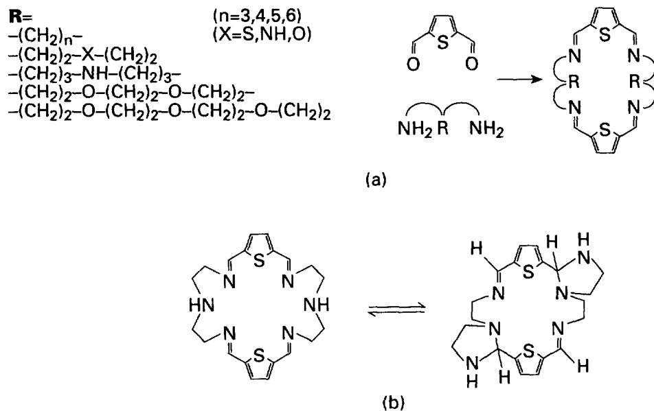
Scheme 14.
