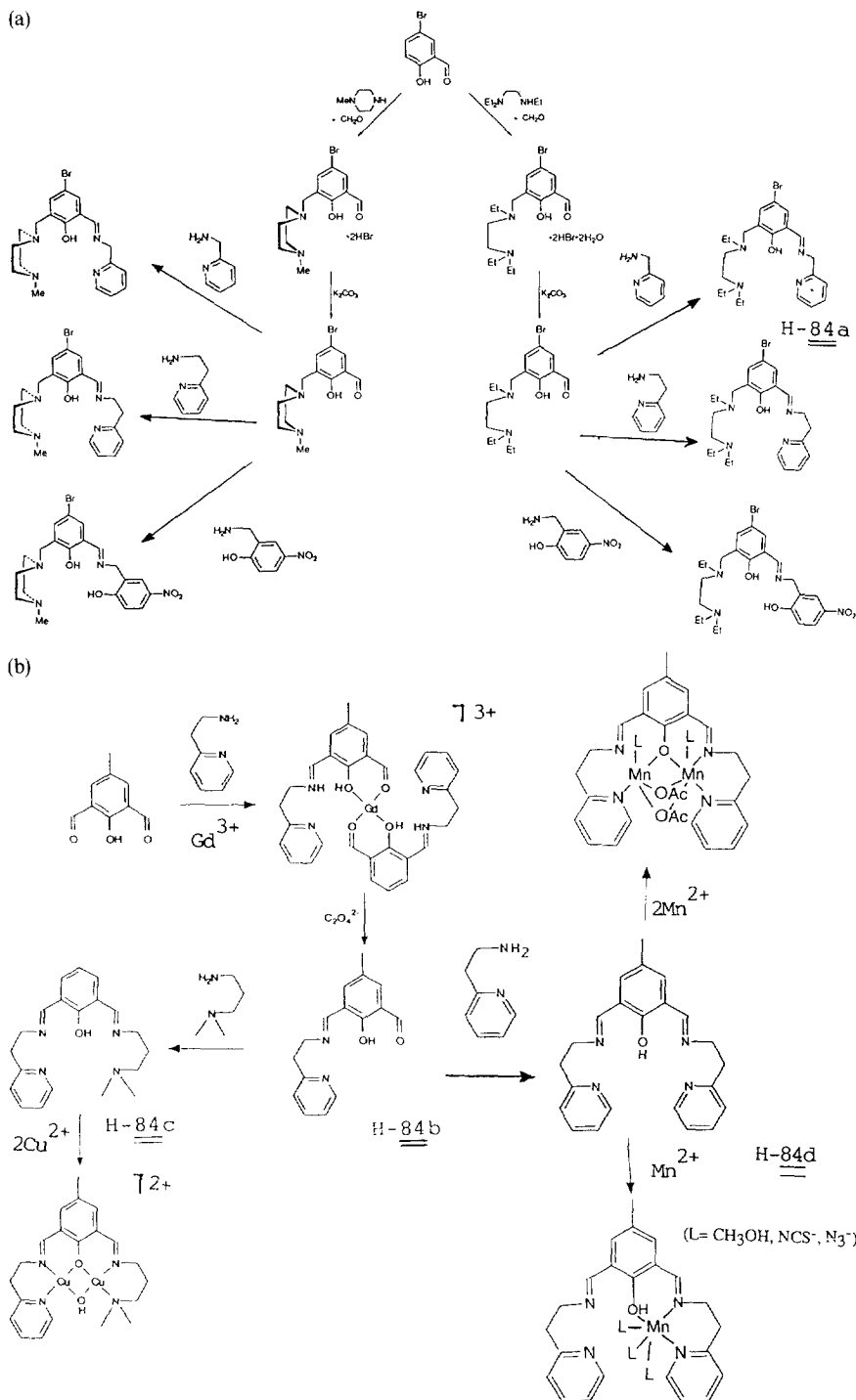
Scheme 29.
