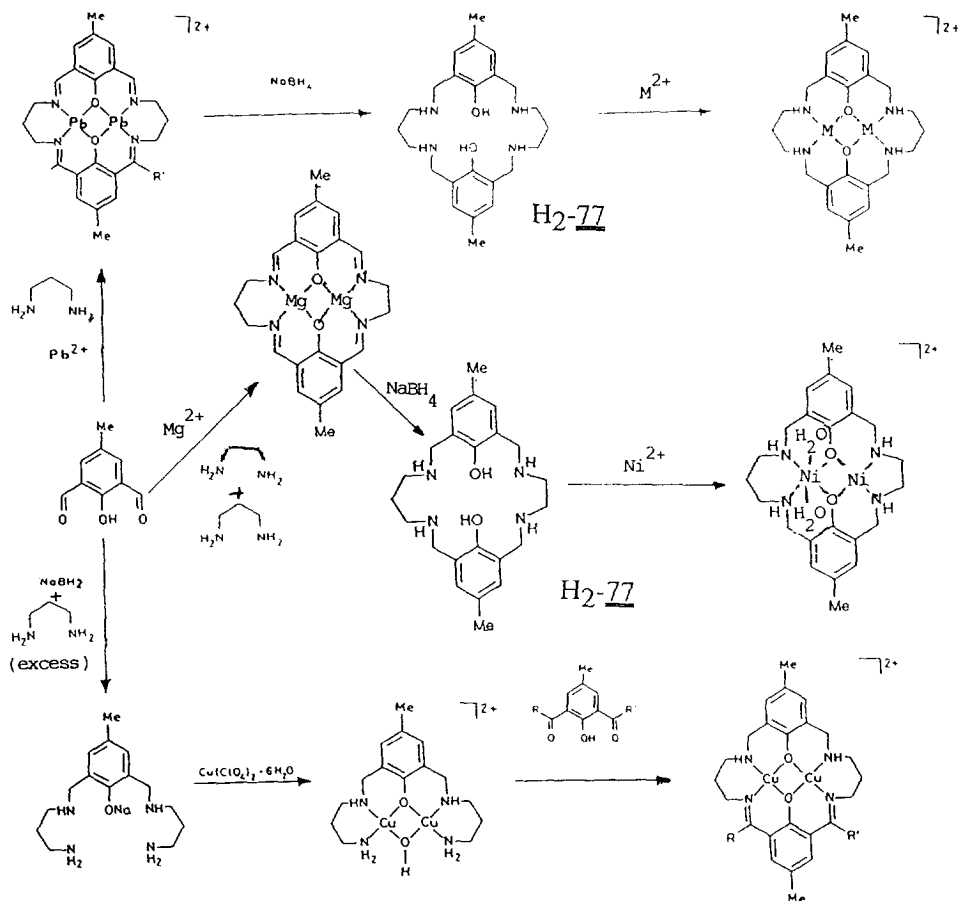
Scheme 27.
