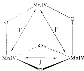
B: Trinuclear
