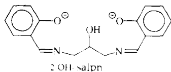
2 OH-salpn
