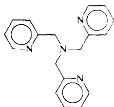
tmpa
