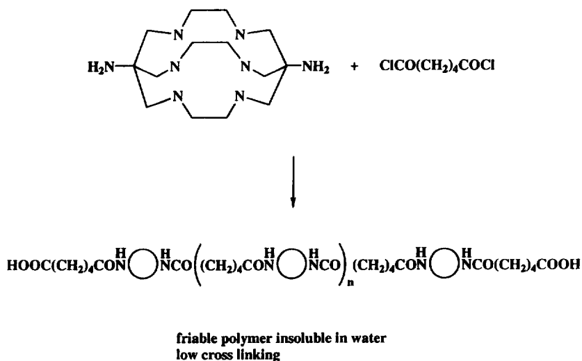
Fig. 10. Cage polymer.
