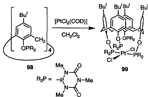
Scheme 21.
