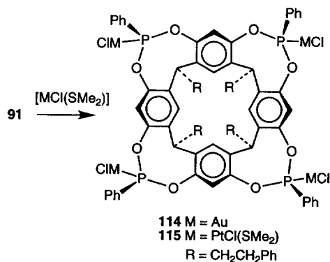
Scheme 25.
