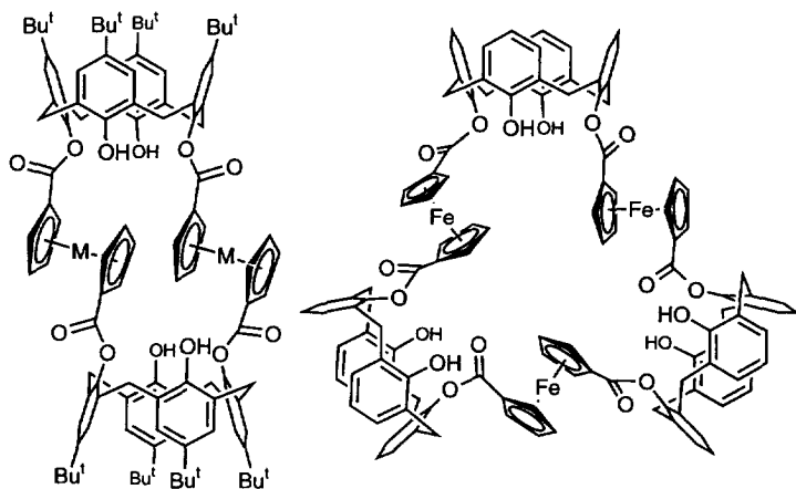
189 M = Fe 190 M = Ru
