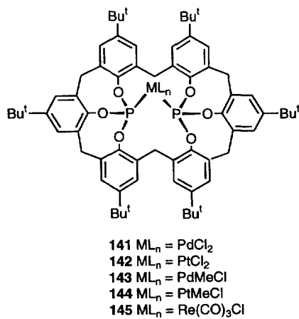
Scheme 31.
