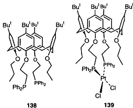
Scheme 30.
