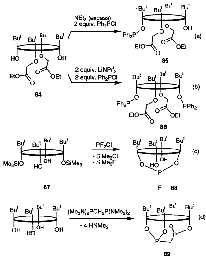
Scheme 18.
