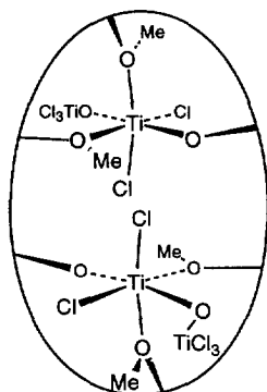
p -tert-butylcalix[6]-(OMe) 4 -(O) 2 [TiCl 2 (μ-O)TiCl 3 ] 2 42
