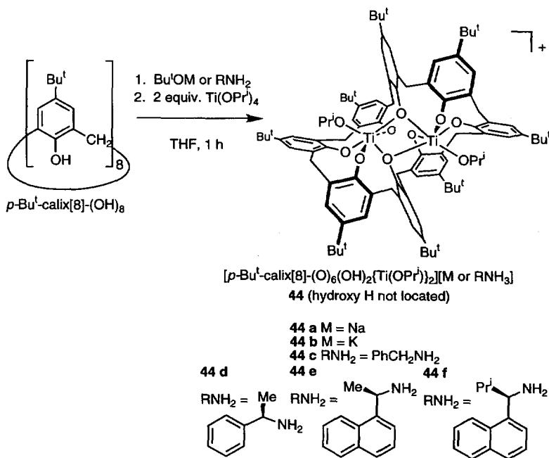
Scheme 14.
