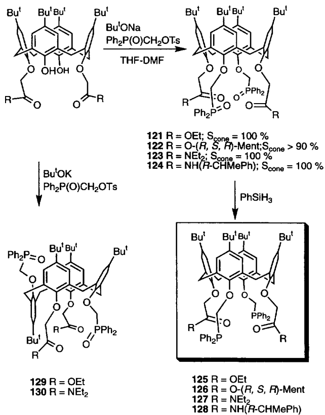
Scheme 28.
