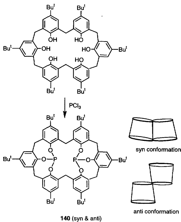
Scheme 31.
