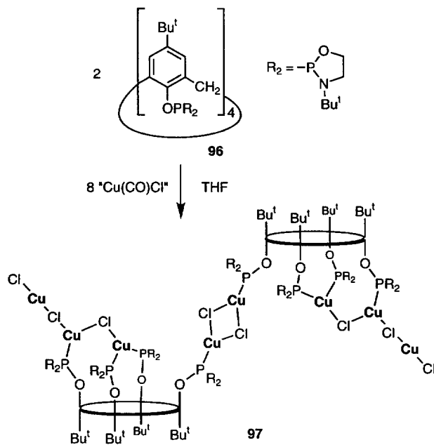
Scheme 20.
