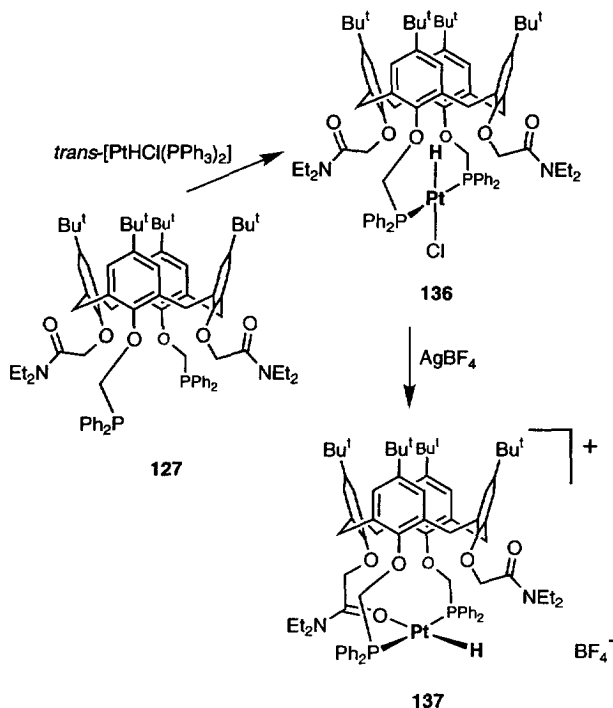
Scheme 30.
