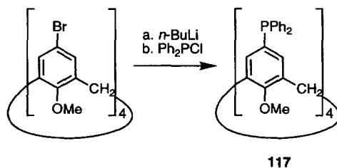
Scheme 26.
