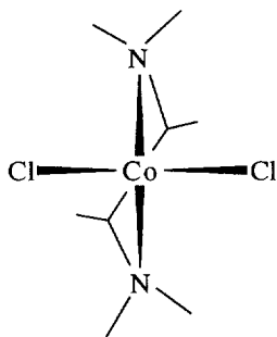
Fig. 34. Chromophore 12 .
