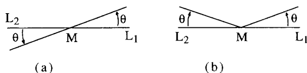
Fig. 20. (a) Gerade and (b) ungerade bending modes.
