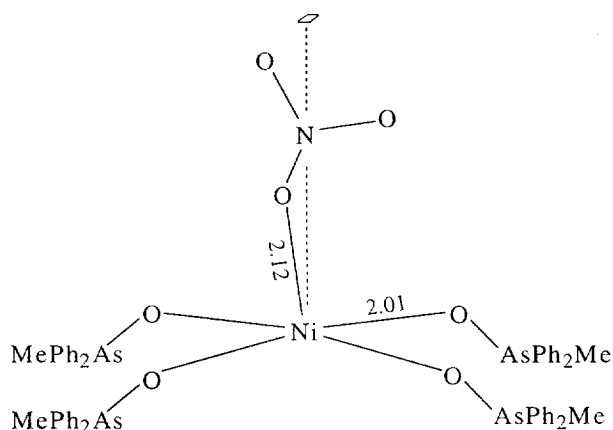
Fig. 33. Chromophore 42 .
