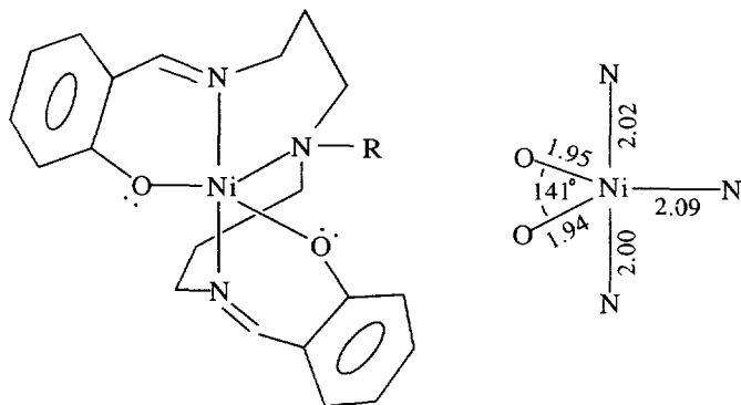
Fig. 32. Chromophore 32 .
