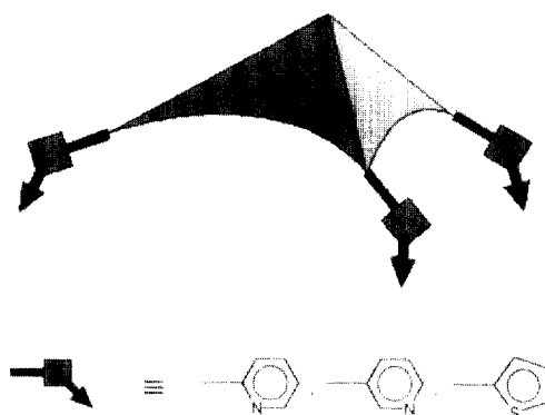
Fig. 11. Side arm donating S(NR)_3 cap.
