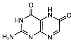
7 xanthoppterin
