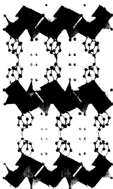
Cu(bpa) 0.5 MoO 4
