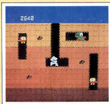
DIGDUG (ATARI)
