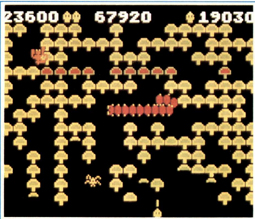
CENTIPEDE (ATARI)
