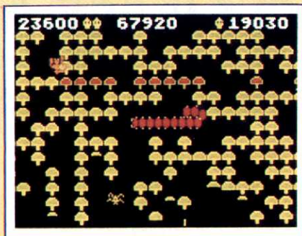
CENTIPEDE (ATARI)
