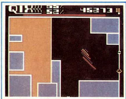
QIX (ATARI)
