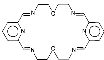
BISBAMP-8H, LH 8 (3)
