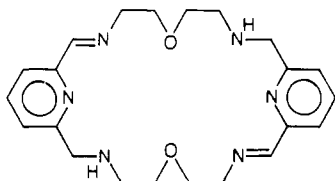
BISBAMP-4H, LH 4 (2)
