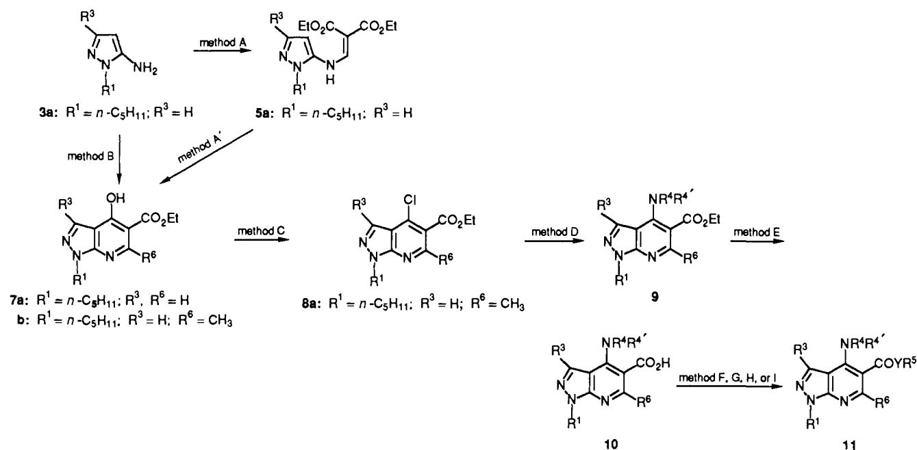
Scheme I a,b
