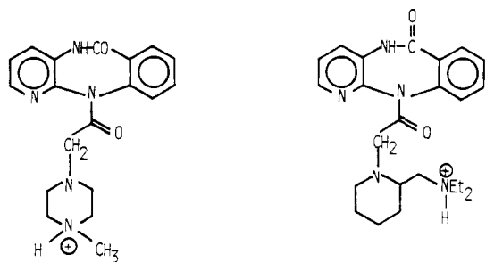
Pirenzepine (1)
