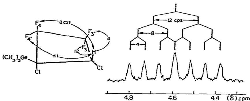
Fig. 3. ^1\text{H} NMR spectrum of (\text{CH}_3)_3\text{GeCCICClHCF}_2\text{CF}_2 .
