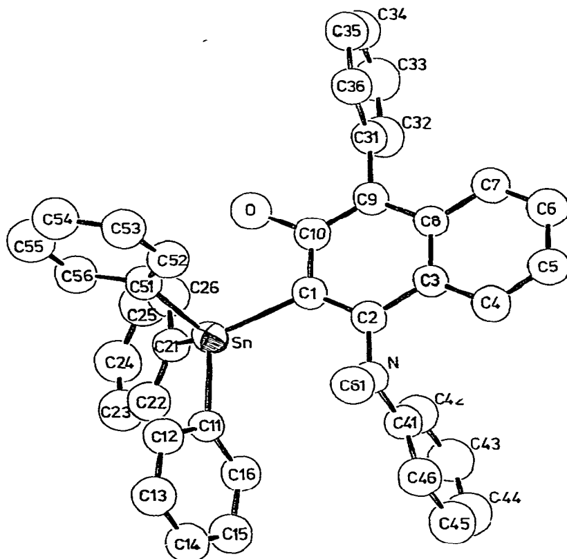
Fig. 1. Molekülstruktur (ORTEP-plot) von 4( N -Methylanilino)-1-phenyl-3-triphenylstannyl-2-naphthol (Xb).
