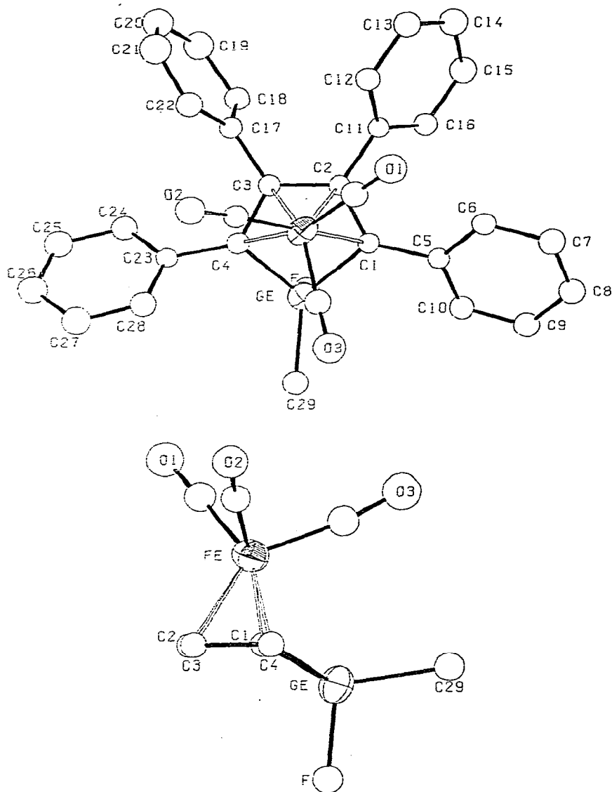
Fig. 1. Molekülstruktur von Tricarbonyl(1- exo -fluor-1-methyl-2,3,4,5-tetraphenyl-1-germacyclopentadien)-eisen.
