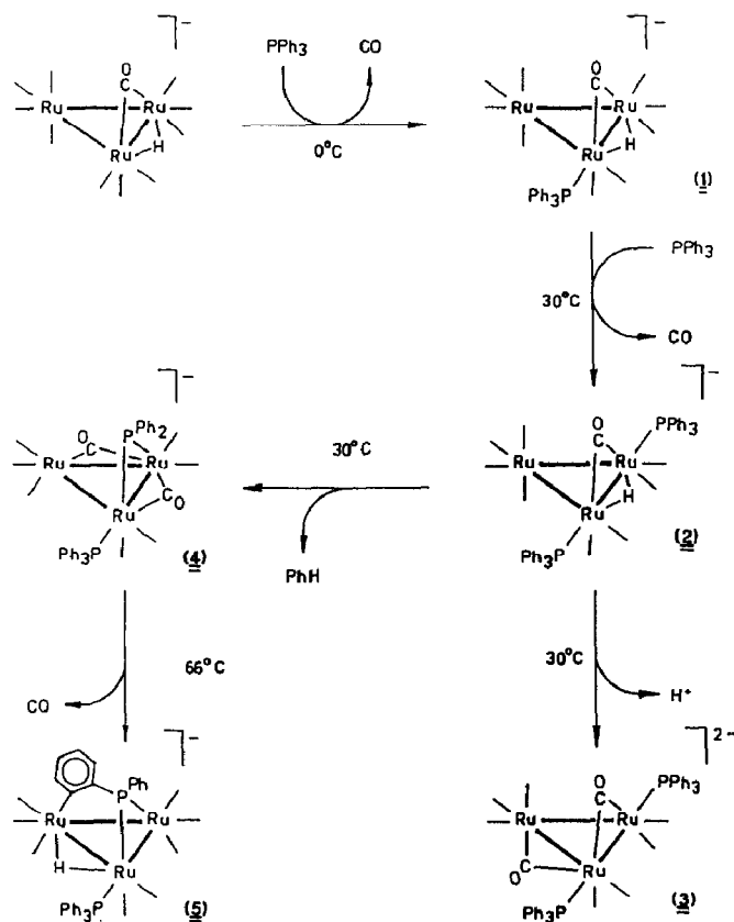
Schema 1. Die Reaktion von [\text{HRu}_3(\text{CO})_{11}]^- mit \text{PPh}_3 in THF-Lösung.
