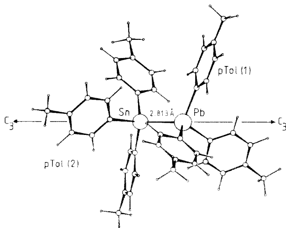
Fig. 3. Gefundenes p\text{-Tol}_6\text{PbSn} -Molekül mit eingezeichneter C_3 -Achse.
