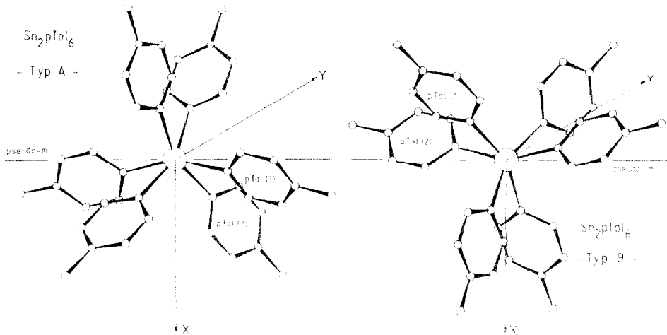
Fig. 2. Typ A (links) und Typ B (rechts) des p\text{-Tol}_6\text{Sn}_2 in Projektion auf die \pi -Ebene mit eingezeichneter Pseudo-Symmetrieebene des Übergangs.
