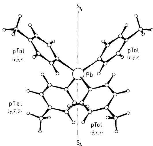
Fig. 1. Gefundenes p\text{-Tol}_4\text{Pb} -Molekül mit eingezeichneter S_4 -Achse und dadurch erzeugten Punktlagen an den vier äquivalenten p\text{-Tol} -Gruppen.
