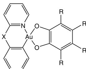
4a , X = NH, R = H 4b , X = CH 2 , R = H 4c , X = NH, R = Cl 4d , X = CH 2 , R = Cl
