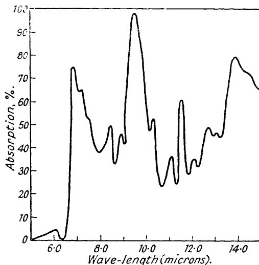
FIG. 1. cis-Hex-3-enol (natural).
