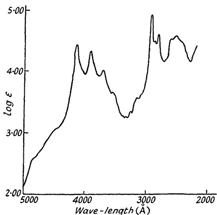
3-Methyl-1 : 2 : 5 : 6-dibenzopyracylene.
