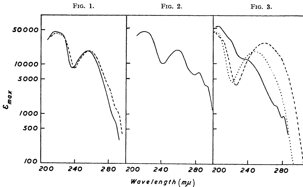
FIG. 1. ——— Methyl 2' : 4' : 1'' : 3''-tetrachloro-3 : 4-5 : 6-dibenzocyclohepta-3 : 5-diene-1-carboxylate (III; R = Me). - - - - 2' : 4' : 1'' : 3''-Tetrachloro-2 : 7-dihydro-3 : 4-5 : 6-dibenzoxepin (I).
