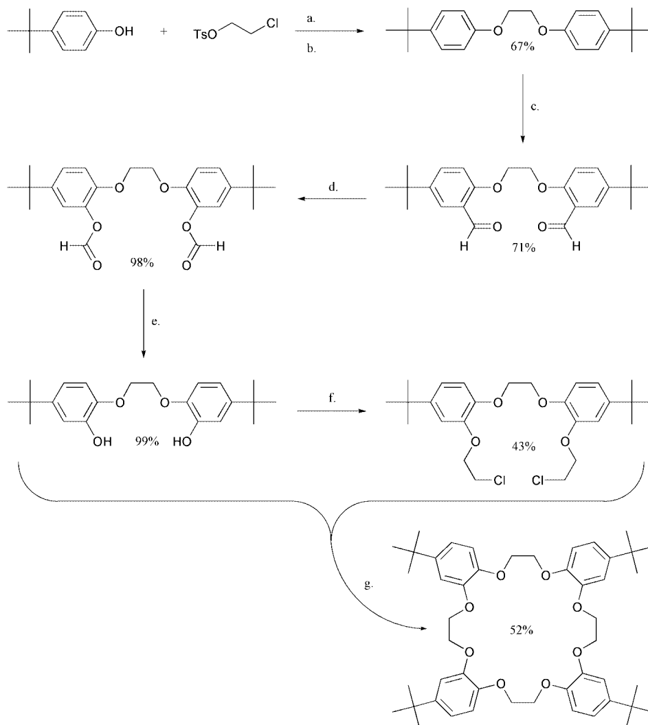
Scheme 1 a. \text{K}_2\text{CO}_3 , \text{CH}_3\text{CN} ; b. \text{KI} , \text{K}_2\text{CO}_3 , \text{DMF} ; c. \text{Cl}_2\text{CHOCH}_3 , \text{TiCl}_4 , \text{CH}_2\text{Cl}_2 ; d. \text{mCPBA} , \text{CH}_2\text{Cl}_2 ; e. (\text{C}_2\text{H}_5)_3\text{N} , \text{CH}_3\text{OH} ; f. \text{TsOCH}_2\text{CH}_2\text{Cl} , \text{K}_2\text{CO}_3 , acetone; g. \text{KI} , \text{Cs}_2\text{CO}_3 , \text{DMF} .
