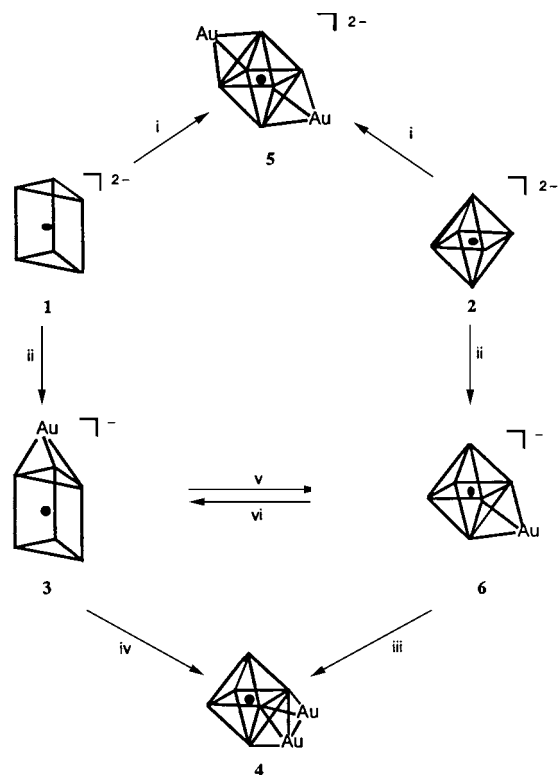
Scheme 1 (i) +2 AuPPh 3 + , RT, acetone; (ii) +AuPPh 3 + , Tl + , -12 °C, CH 2 Cl 2 ; (iii) +AuPPh 3 + , Tl + , -12 °C, CH 2 Cl 2 ; (iv) +2 AuPPh 3 + , Tl + , -12 °C, CH 2 Cl 2 ; (v) heat, CH 2 Cl 2 ; (vi) +CO, -12 °C, CH 2 Cl 2 .
