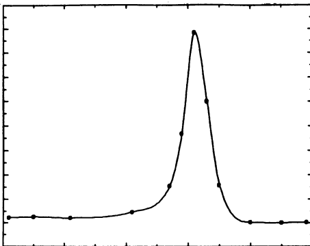
E. CC cubic
