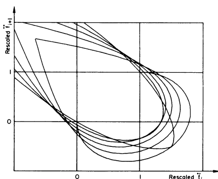
D. \dot{f}_i = \dot{f}_{i+1} , rescaled
