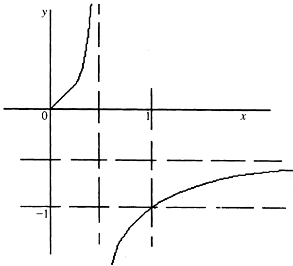
FIGURE 2. y = -x/(2x - 1)
