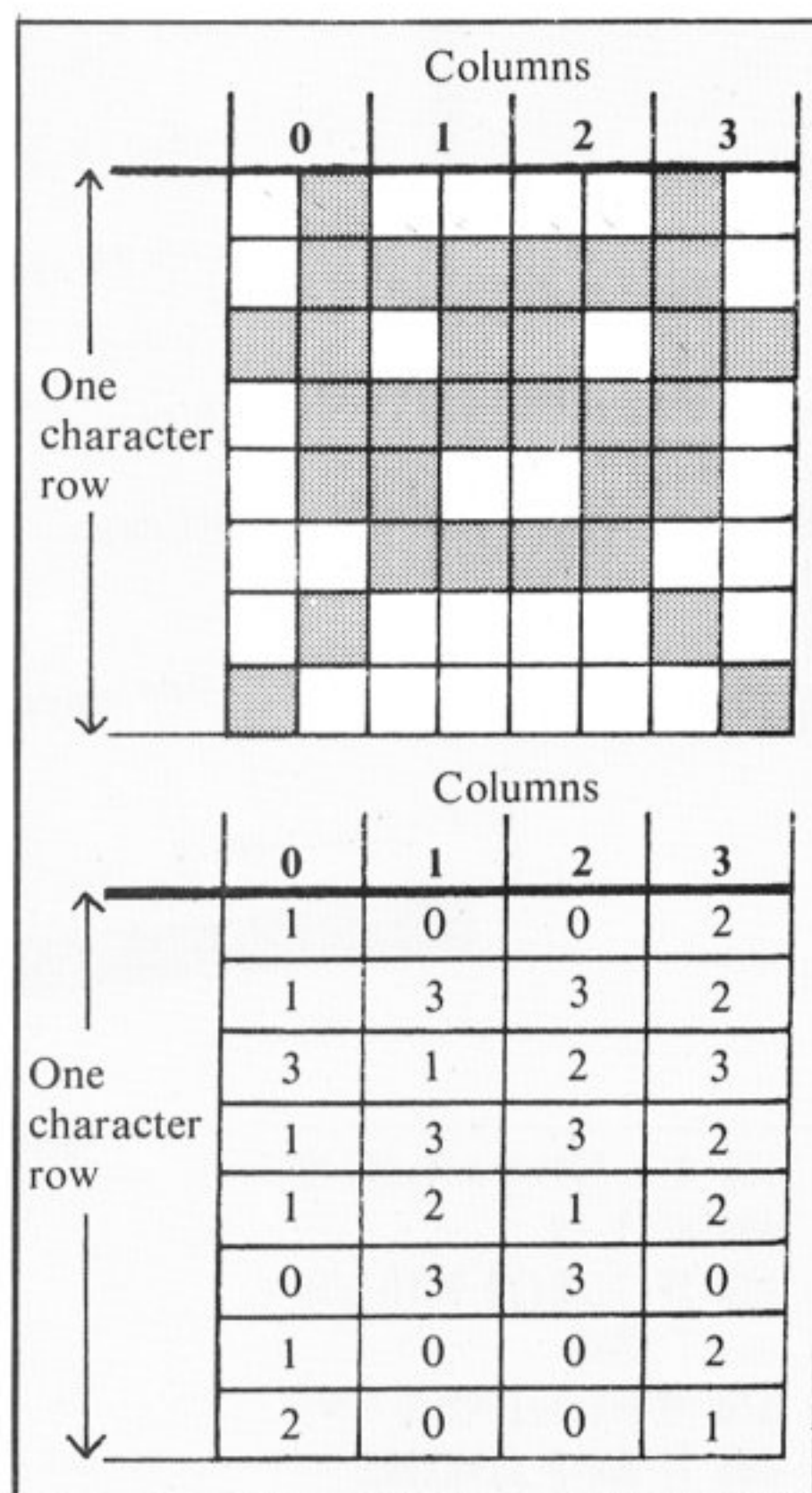
Diagram II: Parameters for a red invader
