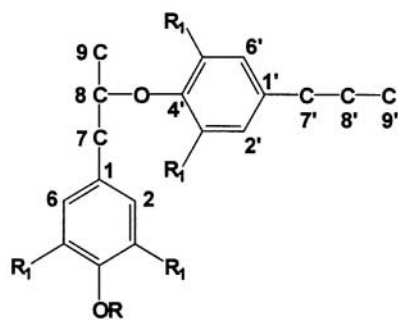
1 R = H or CH 3 R 1 = H or OCH 3
