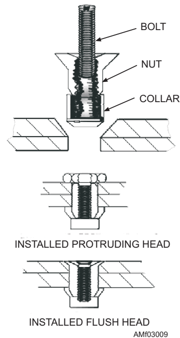
Figure 3-9.—Jo-bolt.
