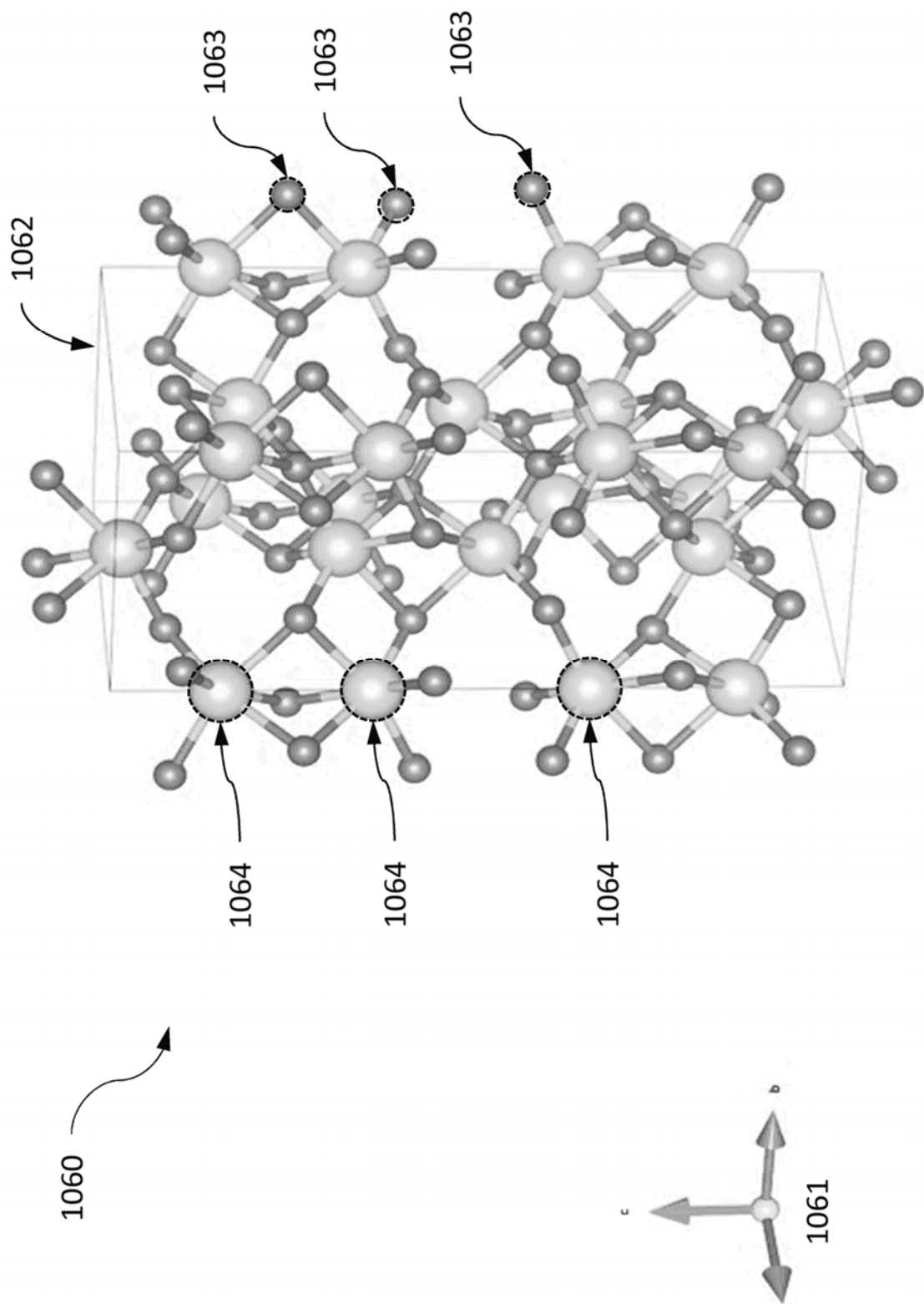
FIG. 31 Al 2 O 3 -trigonal (Corundum)
